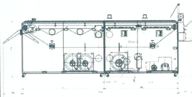
ITS-3000 側面図
